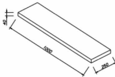
Typ 1000×250×40mm
